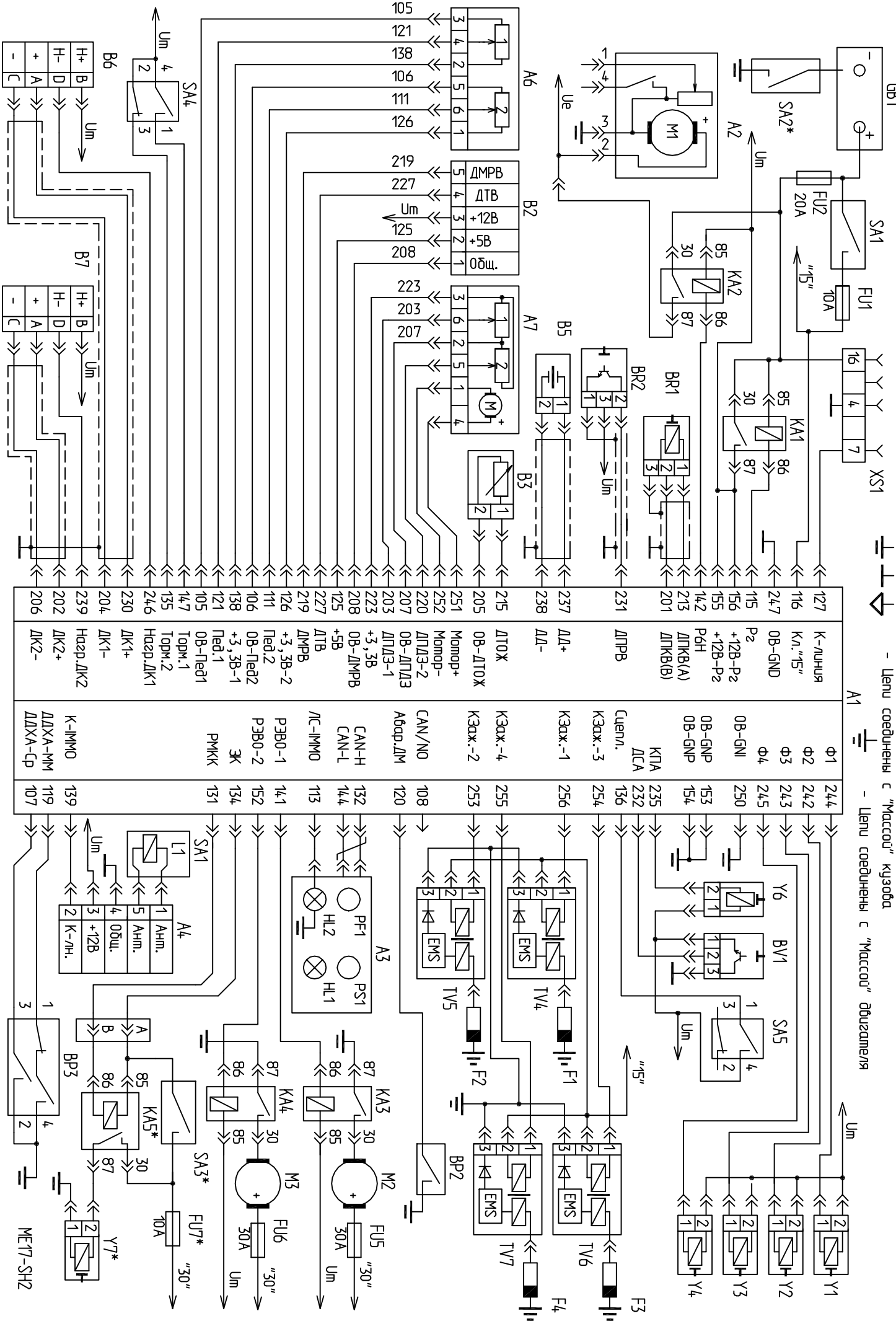
Схема электрическая функциональная ЭСУД с контроллером МЭТ7.9.7/Евро-3 для УАЗ-3163 (ЭМЗ-40904.10)
